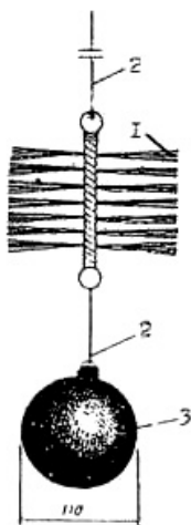
4 pav. Įtaisas dūmtraukio ar ventiliacijos kanalų valymui: 1 – metalinis šepetys, 2 – plieninis troselis, 3 – metalinis rutulys
