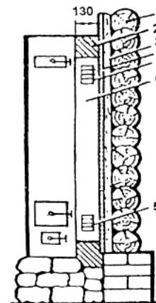
2 pav. Krosnies mūrijimas prie medinės sienos: 1 – medinė siena, 2 – plytų mūrinys, 3 – medinis skydas, 4 – ugniai atspari izoliacinė medžiaga, 5 – ventiliacinės angos, 6 – krosnies atitolinimas, lygus 130 mm
