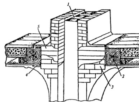
1 pav. Dūmtraukio mūrijimas degioje perdangoje: 1 – dūmų kanalas, 2 – medinis balkis, 3 – dūmtraukio praplatėjimas, 4 – ugniai atspari izoliacinė medžiaga, 5 – dūmtraukio praplatėjimas iki 250 mm
